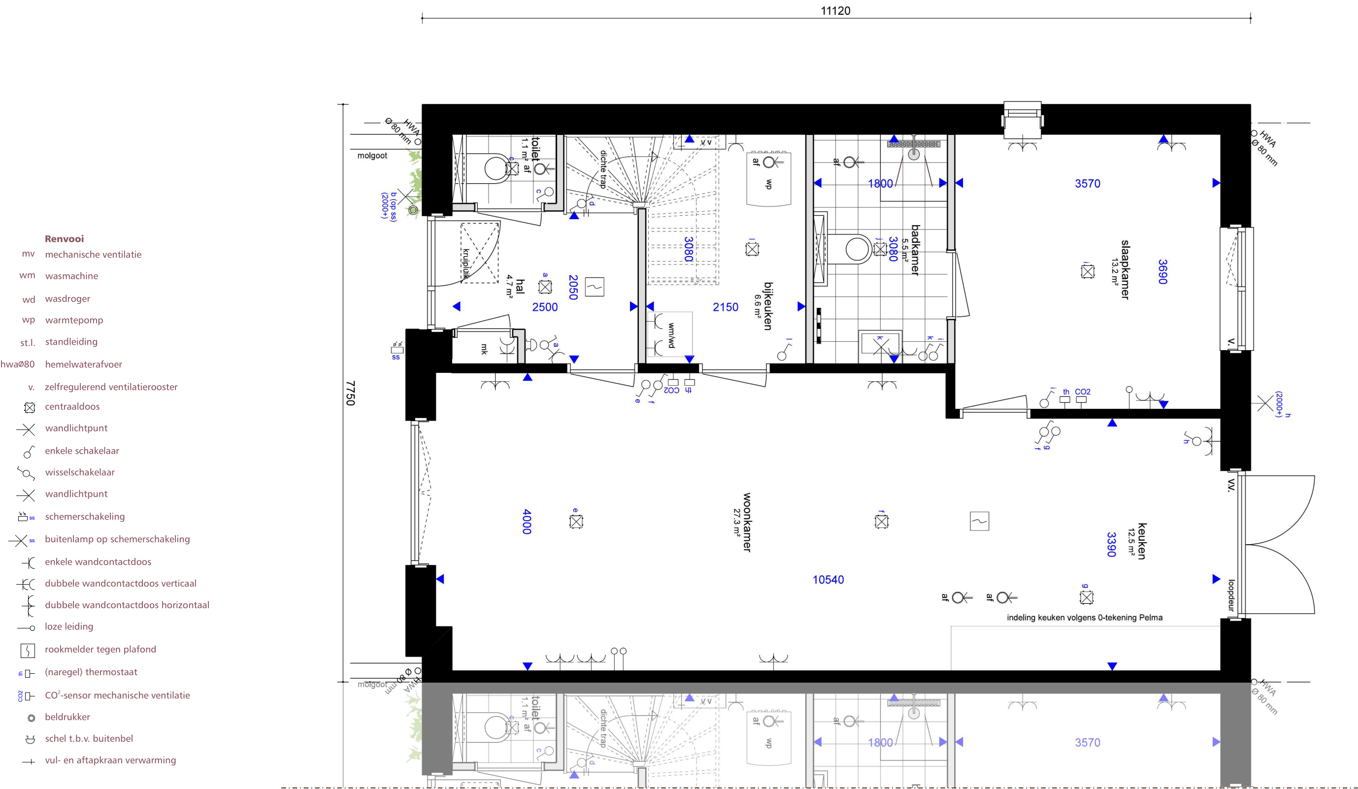
SCHAAL 1 OP 50 Plattegrond ~ Begane grond
